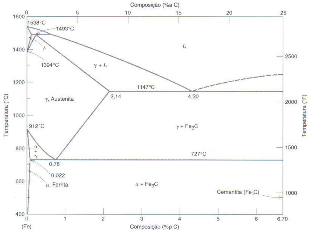
Fig. 9.1. Diagrama de fases do sistema ferro-carbono. (Fonte: Callister e Rethwisch, 2002)
